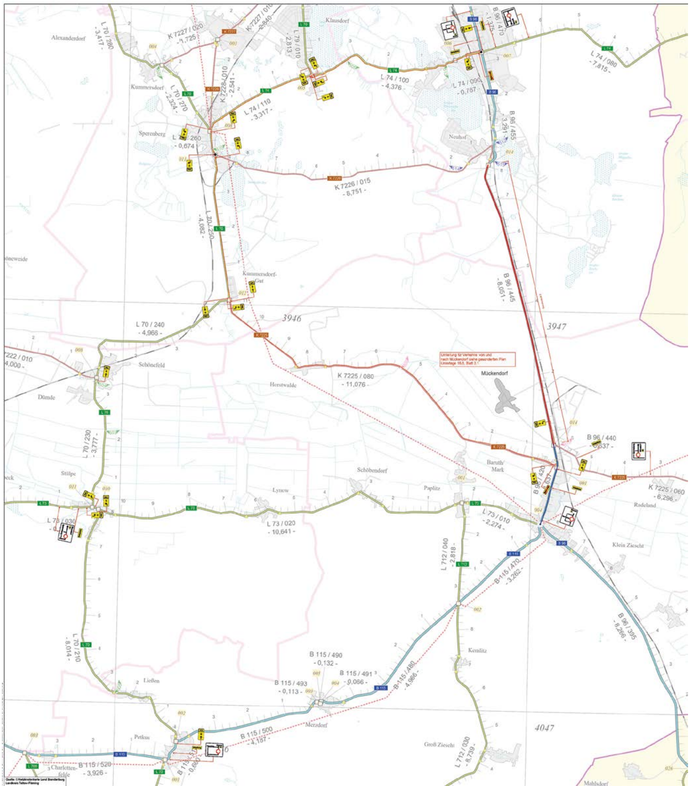
Foto: Umleitungsplan für den 3. Bauabschnitt auf der B 96 nach Neuhoof ab Radeländer Weg
