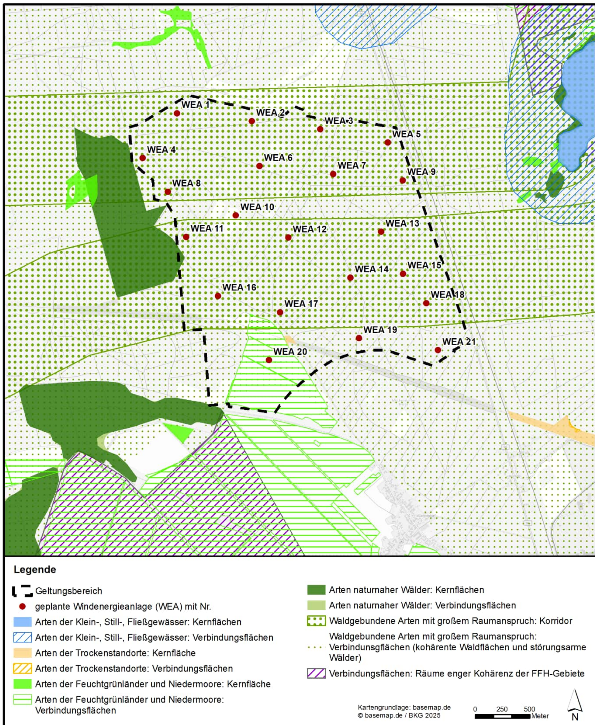
Abbildung 4: Biotopverbundflächen des Entwurfs des Sachlichen Teilplans „Biotopverbund Brandenburg“ des Landschaftsprogramms Brandenburg (2016) mit geplanten WEA im Geltungsbereich
